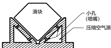
图 10.1: 直线气垫端视图
