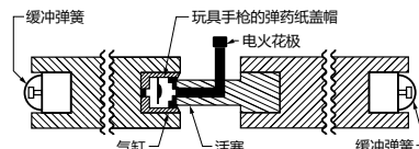
图 10.2: 带有爆破作用气缸附件的滑块截面图
